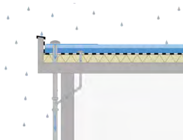
Schematische doorsnede van een regendak bij een normale en een extreme regenbui © Atelier GROENBLAUW
